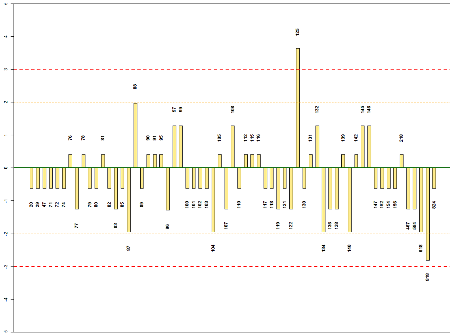
Andamento dei valori di z-score (FdC) - campione 33
