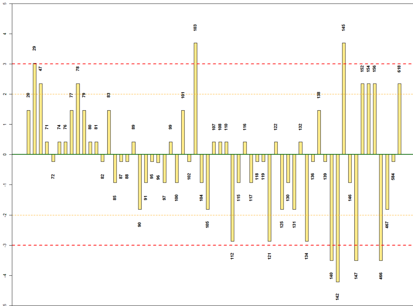
Andamento dei valori di z-score (FdC) - campione 62
