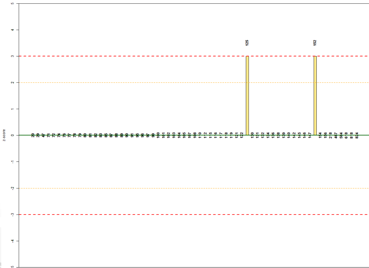
Andamento dei valori di z-score (FdC) - campione 31
