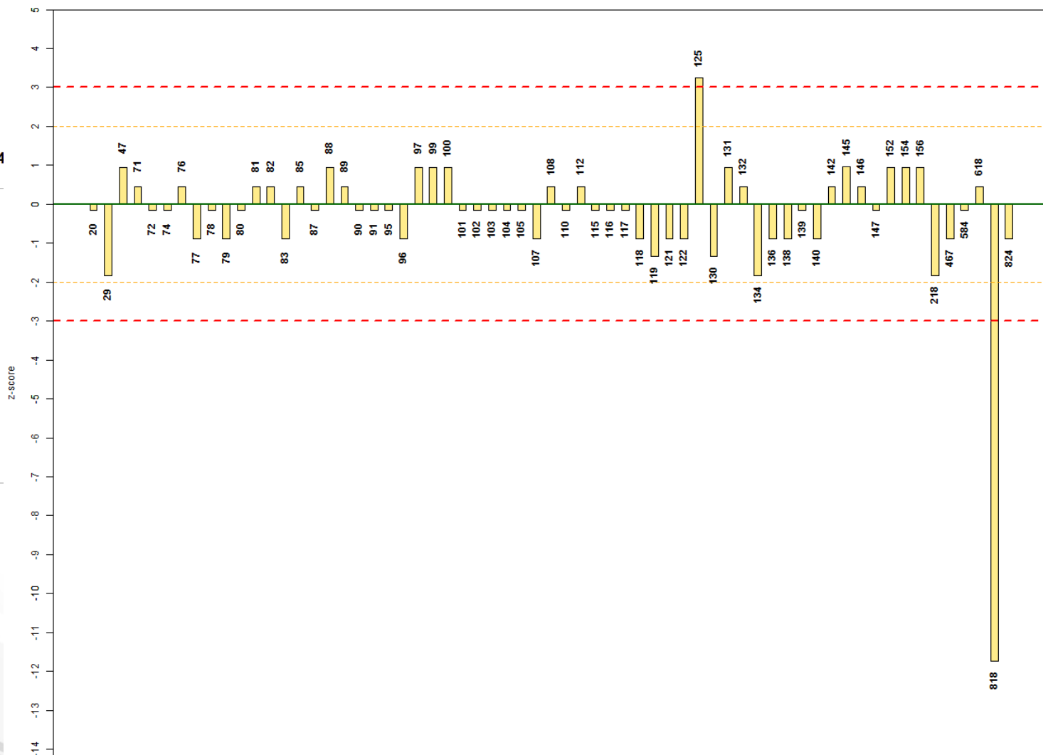
Andamento dei valori di z-score (FdC) - campione 32
