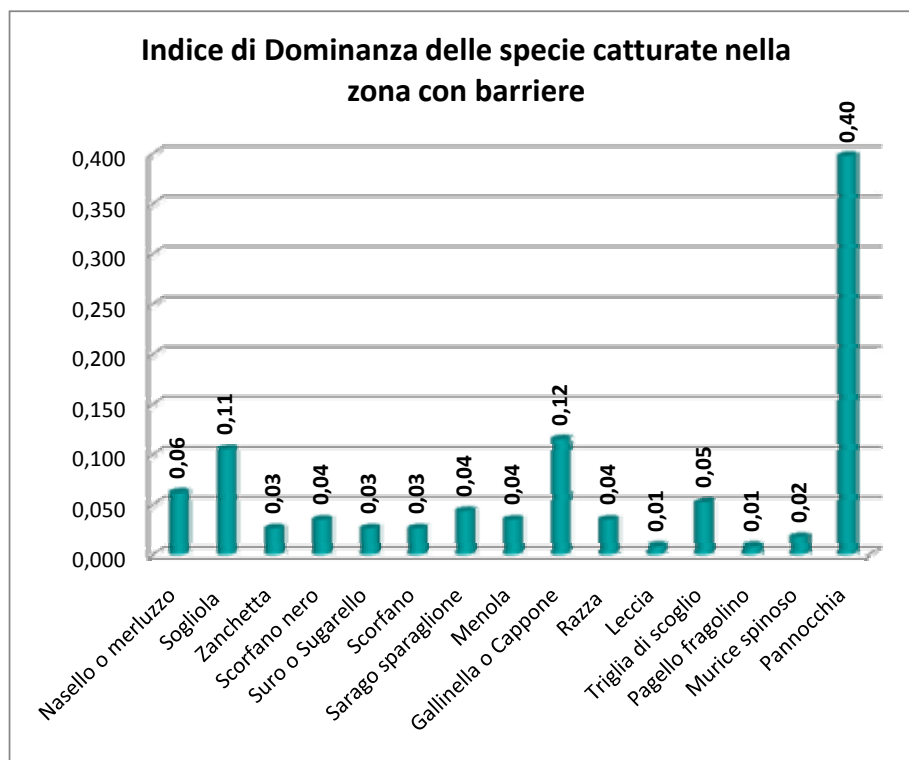
Grafico 21. Indice di Dominanza per il punto di campionamento all'interno della zona con barriere (2009).
