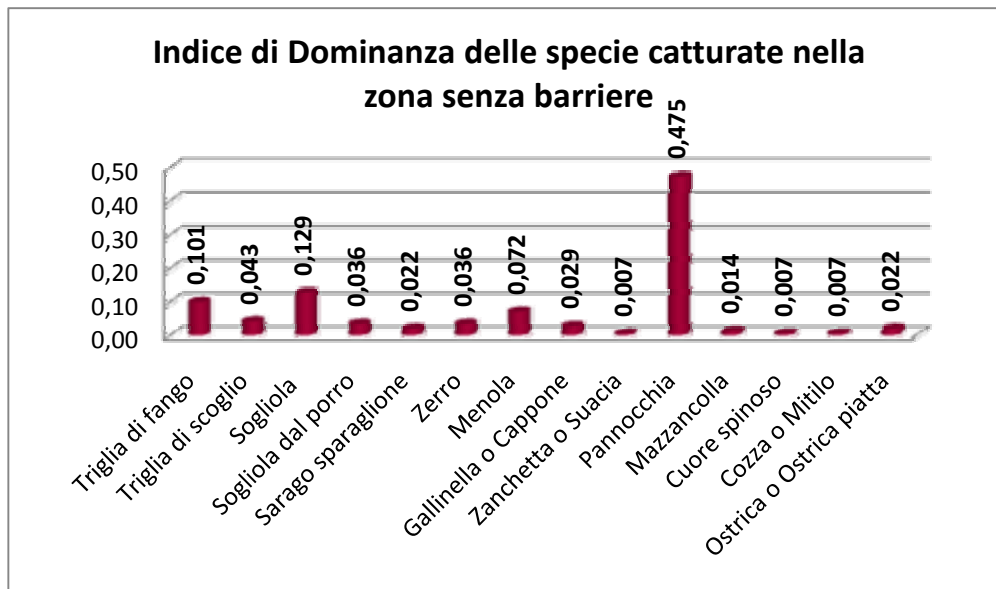
Grafico 18. Indice di Dominanza per il punto di campionamento fuori della zona con barriere (ANNO 2007).
