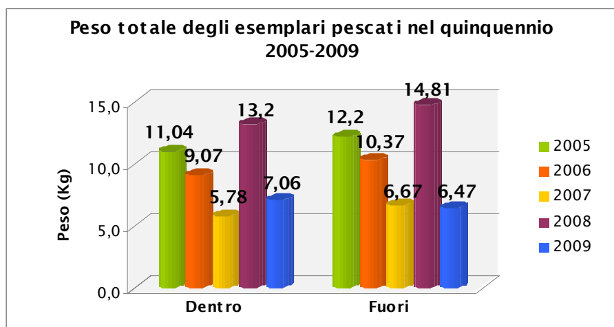
Grafico 11. Peso totale degli esemplari catturati per ciascun punto di campionamento nel quinquennio 2005-2009.
