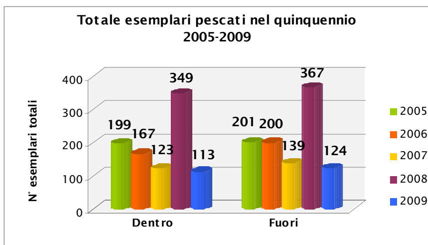
Grafico 10. Numero di esemplari catturati per ciascun punto di campionamento nel quinquennio 2005 - 2009.
