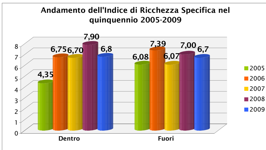
Grafico 12. Ricchezza Specifica per ciascun punto di campionamento nel quinquennio 2005-2009.
