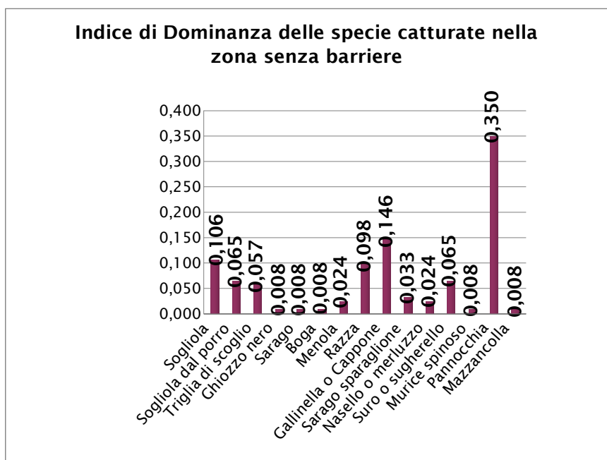
Grafico 7. Indice di Dominanza per il punto di campionamento fuori della zona con barriere.
