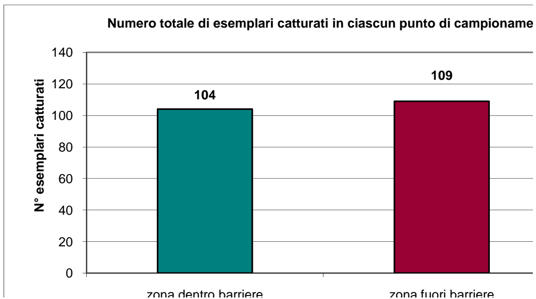
Grafico 3. Numero totale di esemplari catturati nei tre campionamenti nella zona dentro e fuori delle barriere artificiali.
