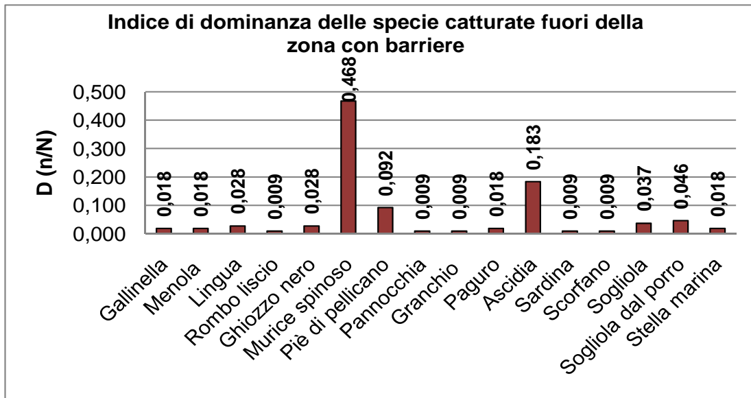
Grafico 9. Indice di dominanza per il punto di campionamento della zona fuori delle barriere artificiali.
