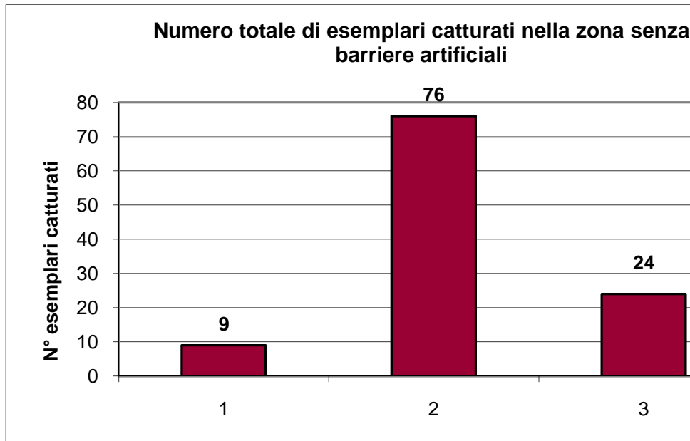
Grafico 2. Numero totale di esemplari catturati nei tre campionamenti nel punto situato fuori della zona con barriere.
