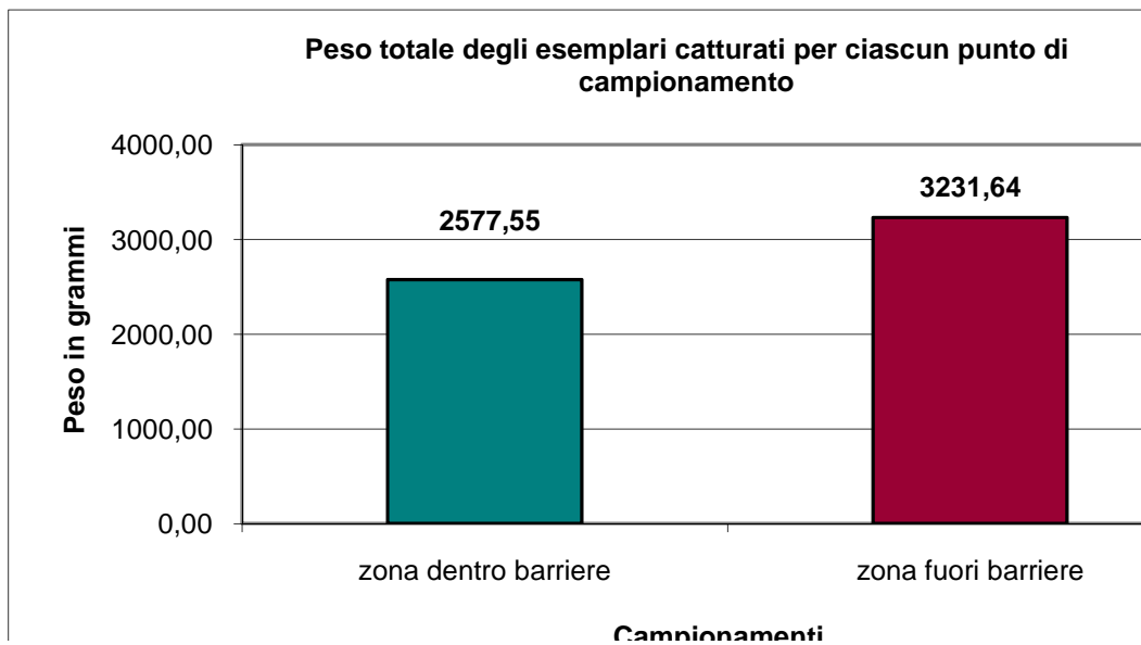
Grafico 6. Peso totale degli esemplari catturati nei 3 campionamenti in ciascun punto di campionamento.
