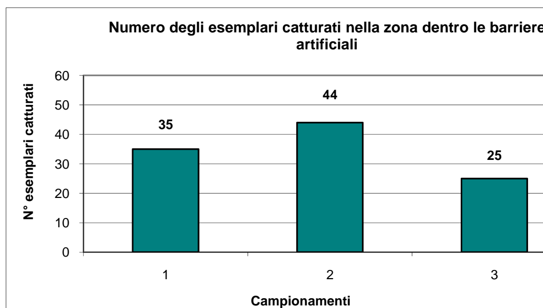
Grafico 1. Numero totale di esemplari catturati nei tre campionamenti nella zona dentro le barriere artificiali.
