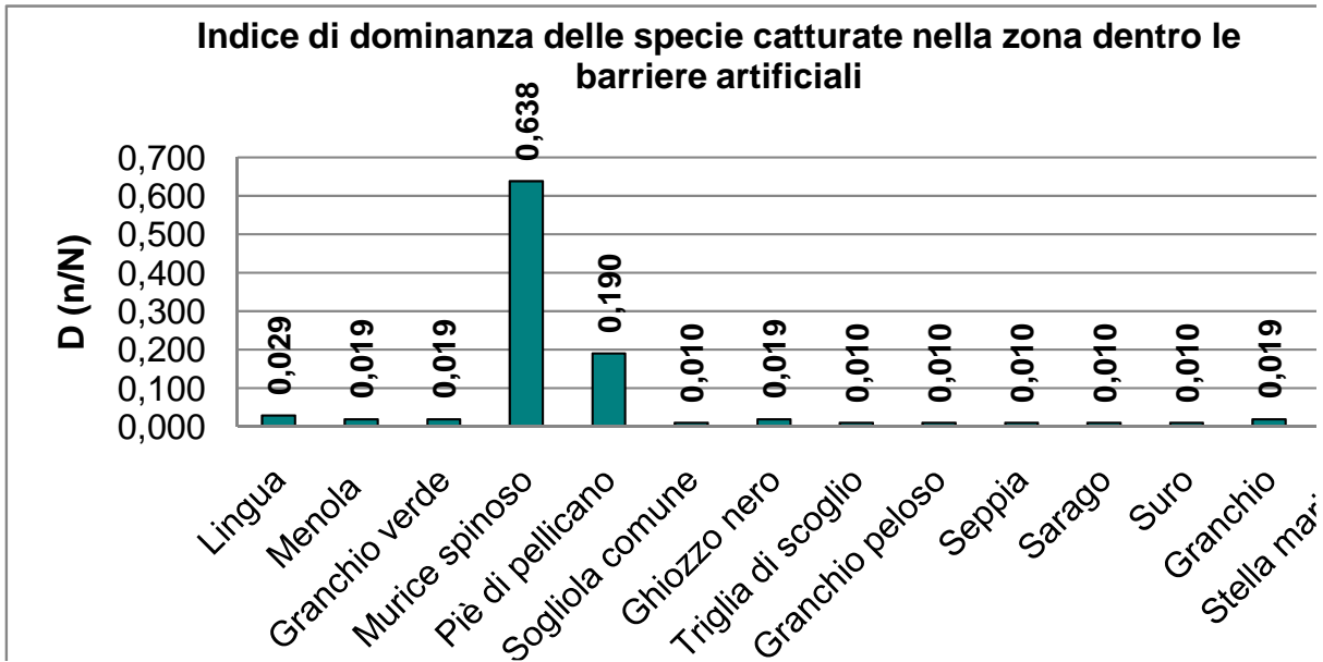
Grafico 8. Indice di dominanza per il punto di campionamento della zona dentro le barriere artificiali.
