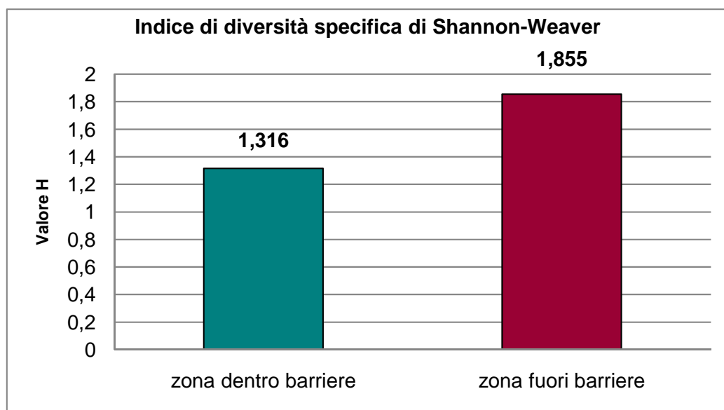
Grafico 10. Indice di diversità specifica di Shannon-Weaver per i due punti di campionamento.
