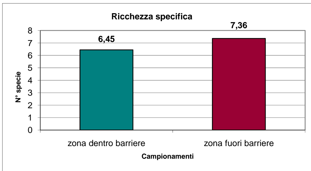
Grafico 7. Ricchezza specifica per ciascuno dei due punti di campionamento.
